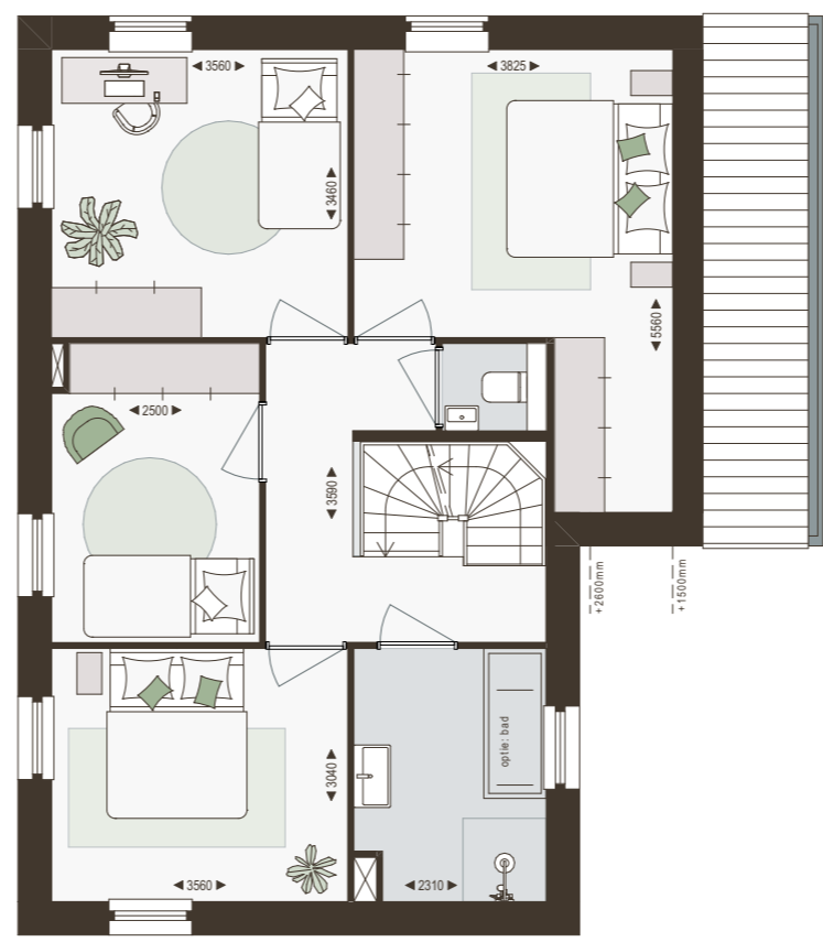
1e verdieping 1:100
